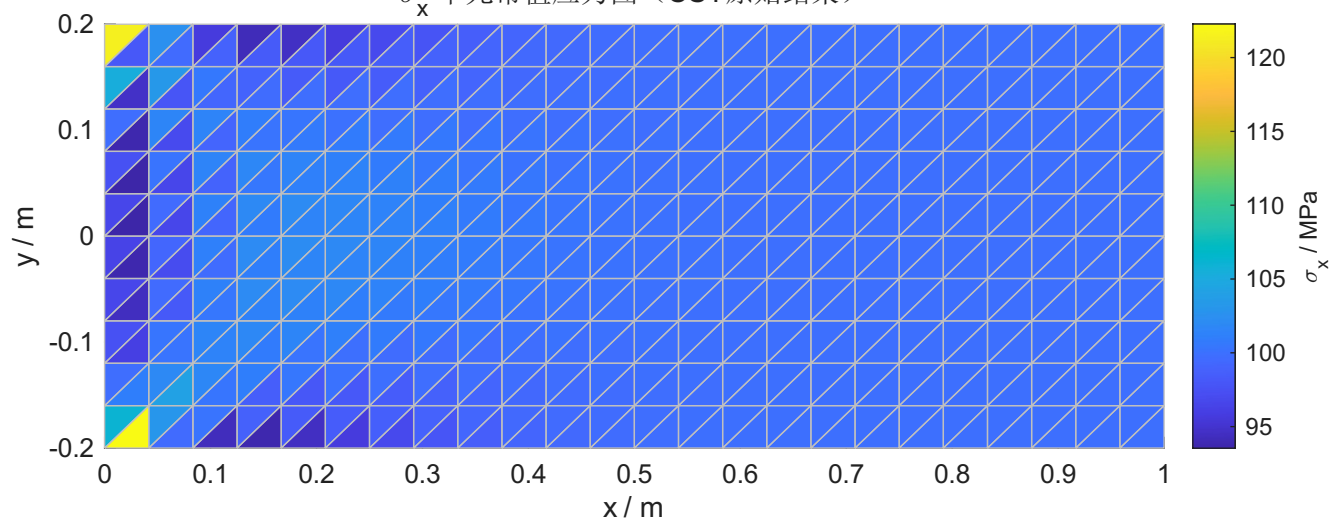
\sigma_x 单元常值应力图 (CST原始结果)
